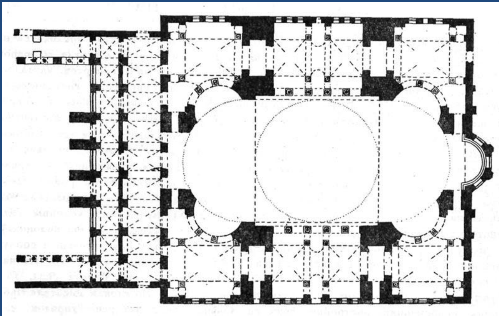
План храма Св. Софии в Константинополе.
