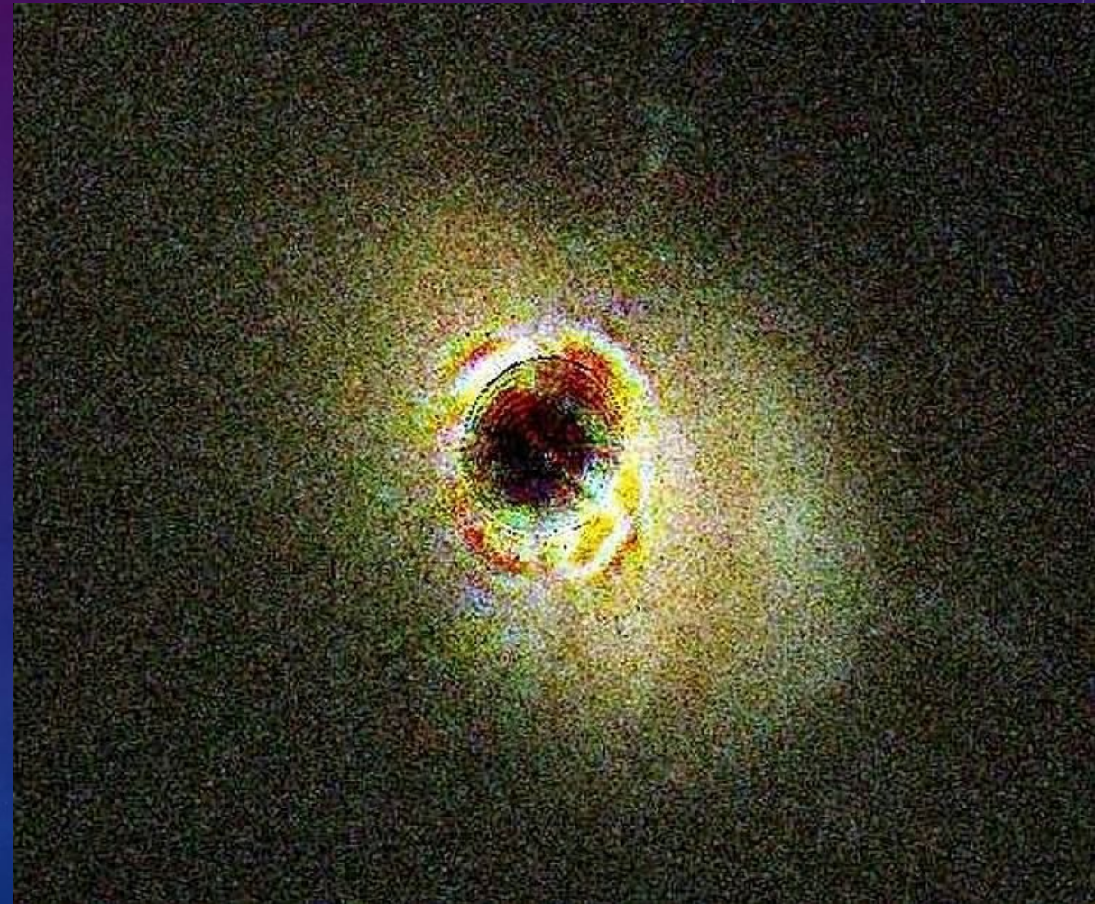
Снимок квазара радиотелескопом
