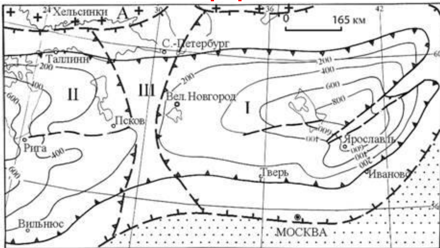
Палеотектоническая карта центра Восточно-Европейской платформы. Каледонский этап . А – Балтийский щит; синеклизы: I – Московская, II – Балтийская; III – Лужская седловина.
