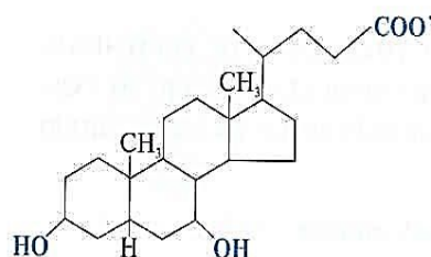
Хенодезоксихолевая кислота
