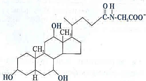
Гликохолевая кислота
