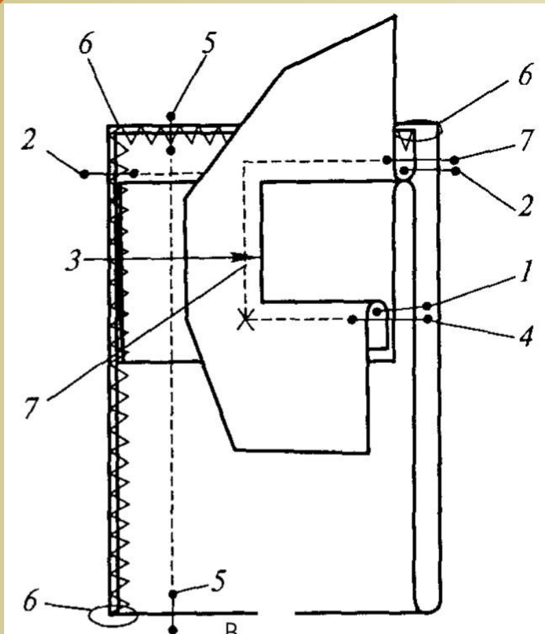
Buzunar tăiat cu laist montat (punga croită integral cu laistul)
