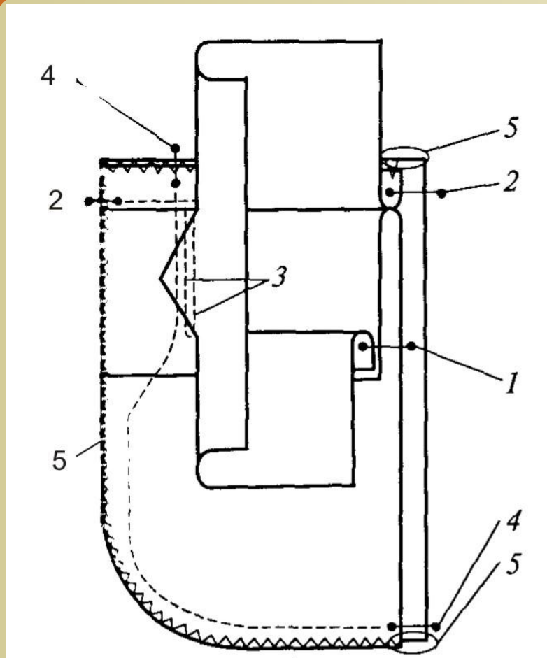
Buzunar tăiat cu laist montat (punga croită integral cu laistul)
