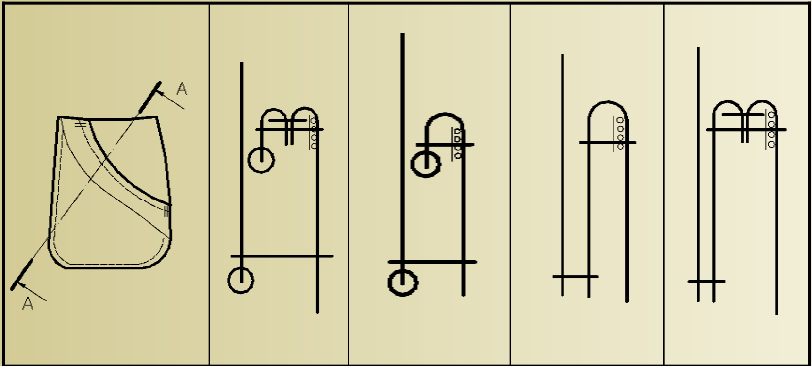
Variante de realizare a buzunarului lateral cu punga din material de bază
