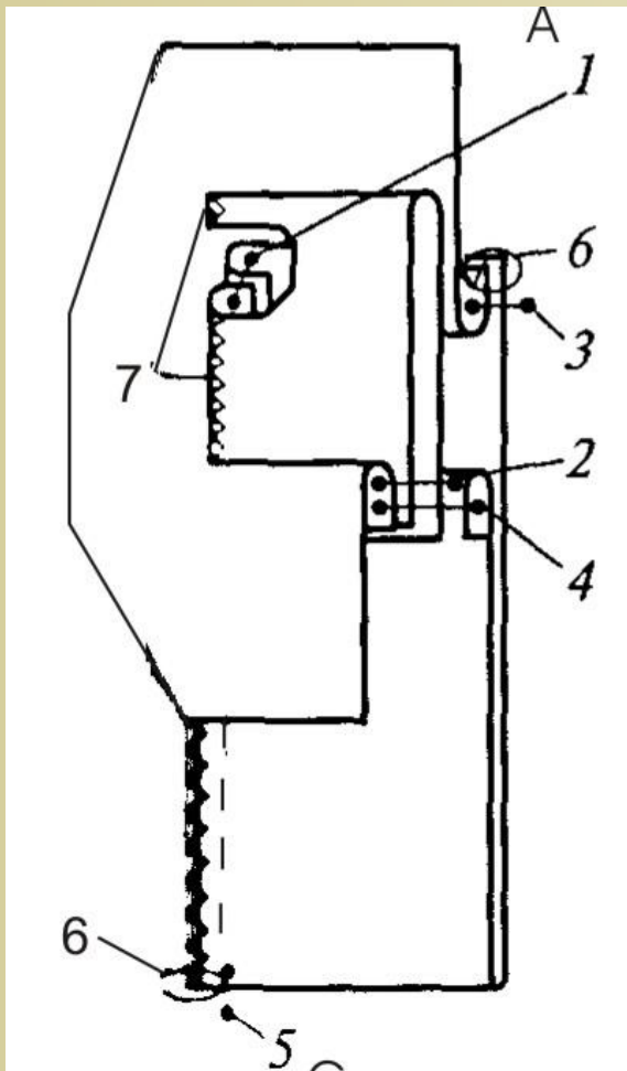
Buzunar tăiat cu laist aplicat (punga croită dintr-un detaliu)
