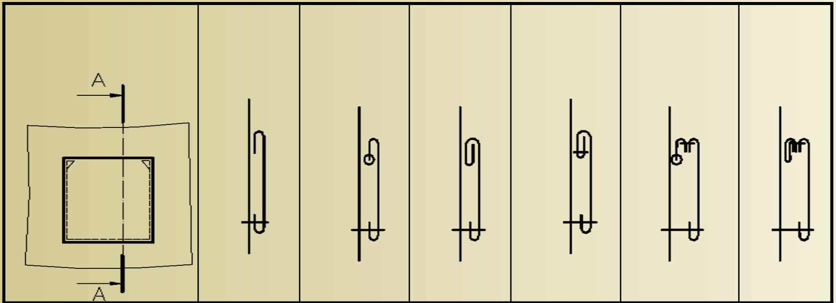
Buzunare aplicate cu rezerva deschiderii fixată în interior
