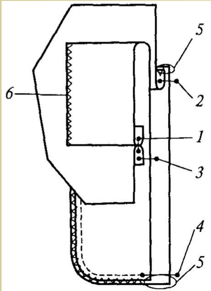
Buzunar tăiat cu laist aplicat (punga croită integral cu laistul)
