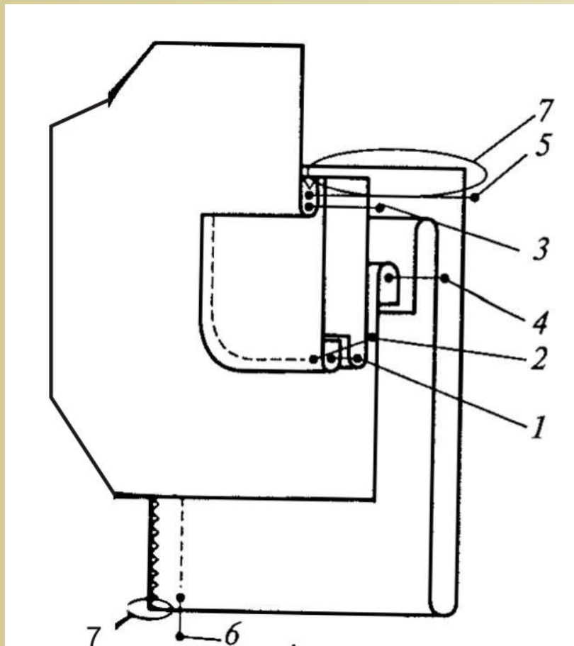
Buzunar tăiat cu clapă și refilet inferior (punga croită integral cu refiletul inferior)
