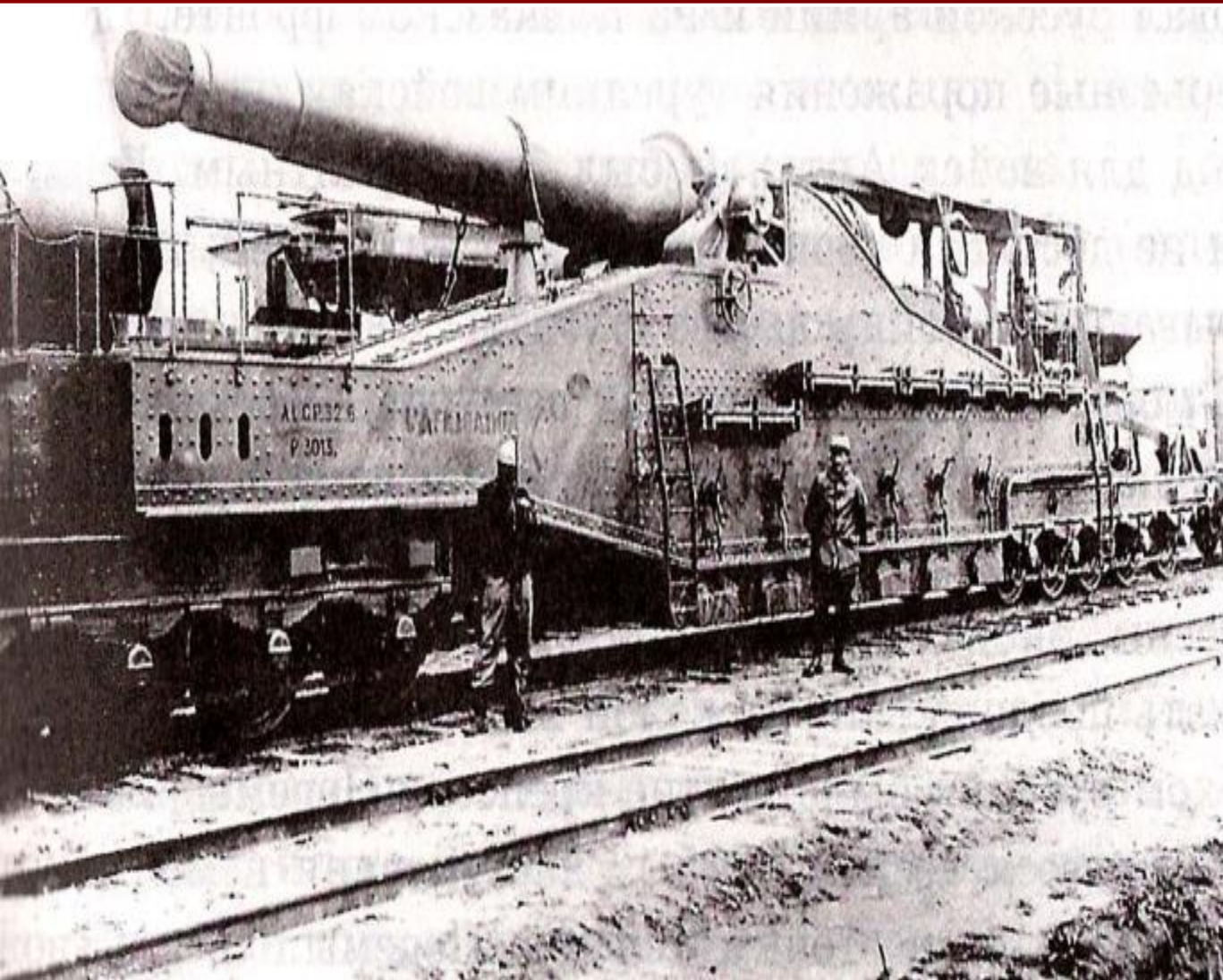
Тяжелое артиллерийское орудие на железнодорожной платформе
