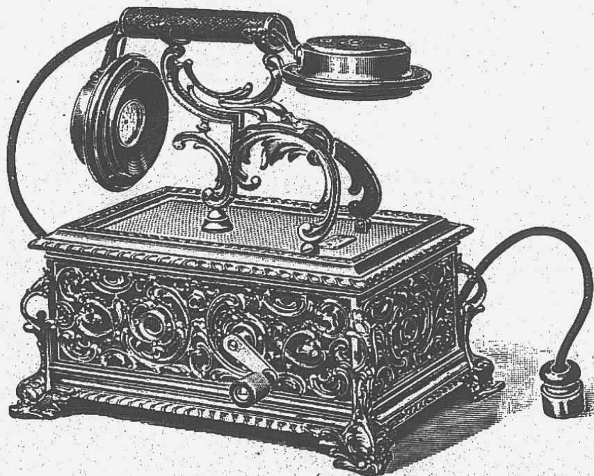
FIG. 109. — Poste téléphonique portatif Siemens et Halske.
