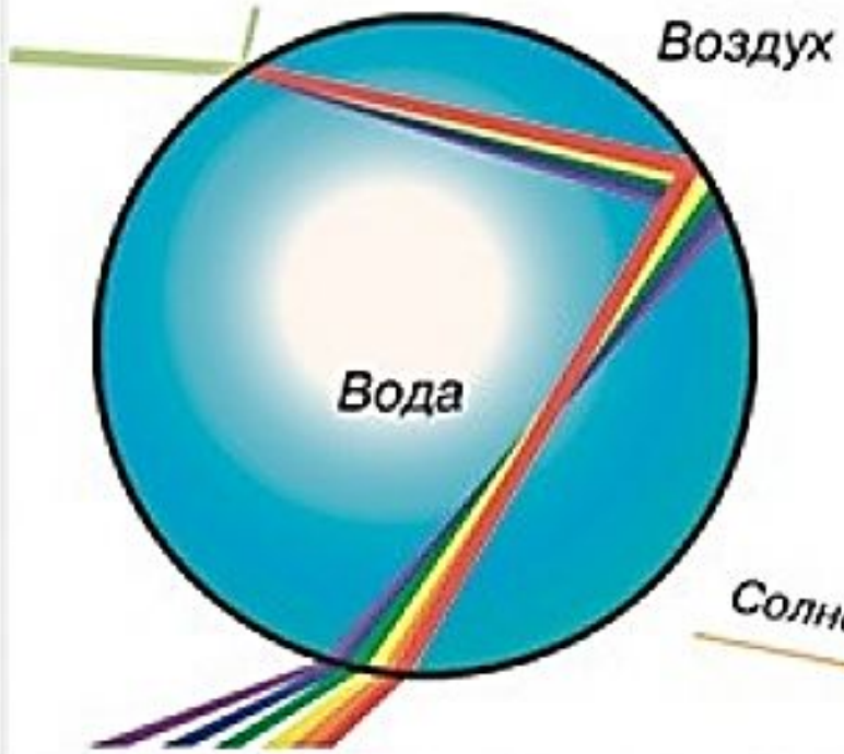
Преломление света в капле воды
