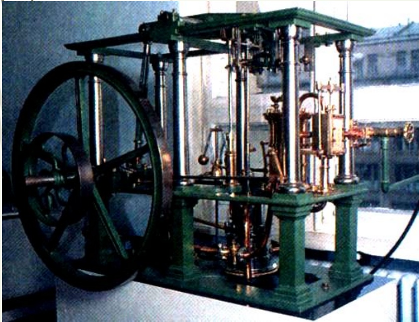
Паровая машина Дж.Уатта
