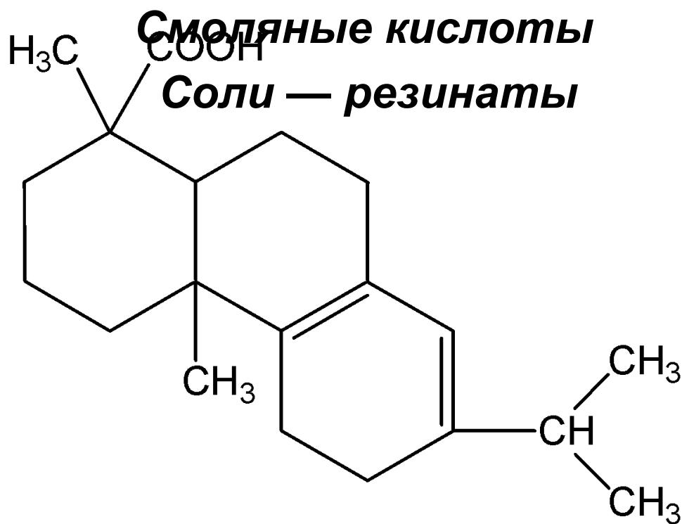
Абиетиновая кислота, C 20 H 30 O 2
