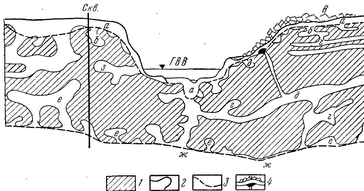
Рис. 109. Схема взаиморасположения мерзлых и талых пород и взаимосвязи над-, меж- и подмерзлотных вод (схематизировано по Н. А. Вельминой): а — надмерзлотные воды; б — надмерзотно-межмерзлотные воды; в — воды криогенных образований; г — межмерзлотные воды; д — межмерзлотные (внутримерзлотные) мощные водоносные горизонты; е — подмерзотно-межмерзлотные воды; ж — подмерзлотные воды; з — «регулирующие подземные резервуары». 1 — мерзлые породы; 2 — талые породы; 3 — нижняя граница надмерзлотных и верхняя подмерзлотных вод; 4 — криогенные образования
