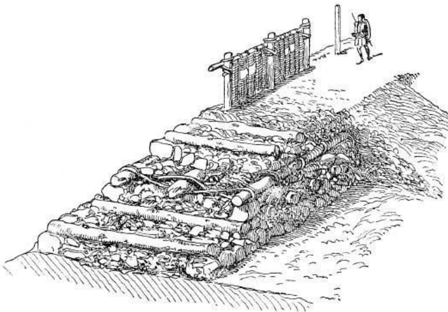
Гальская стена – murus gallicus
