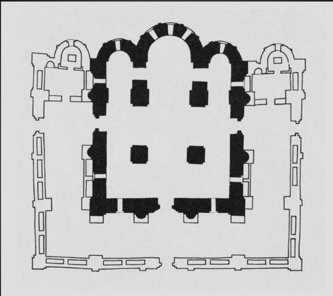
Церковь Иоанна Богослова. Смоленск. 70-е гг. XII в. План.
