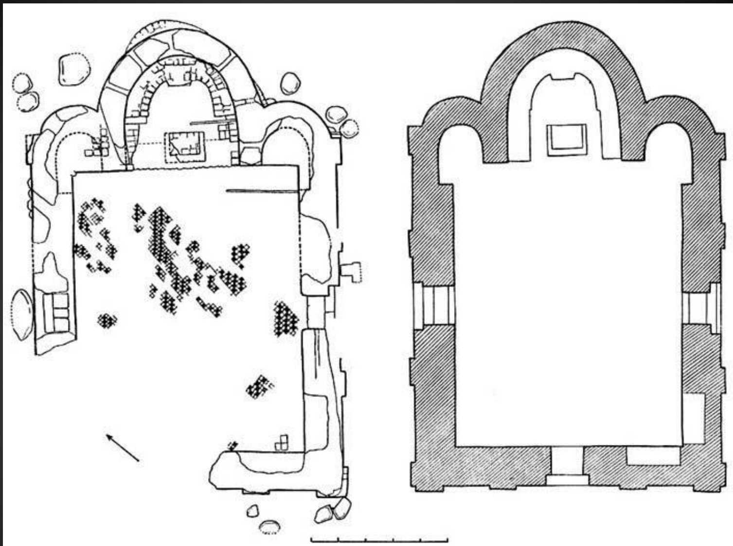
Бесстолпная церковь в детинце. Смоленск. План раскопанного здания и реконструкция плана. Н.Н. Воронин, П.А.Раппопорт
