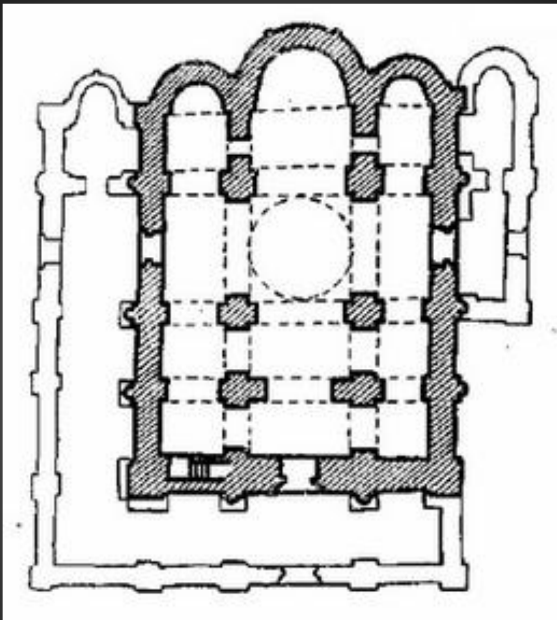
Борисоглебский собор. Чернигов. 20-е гг. XII в. План.
