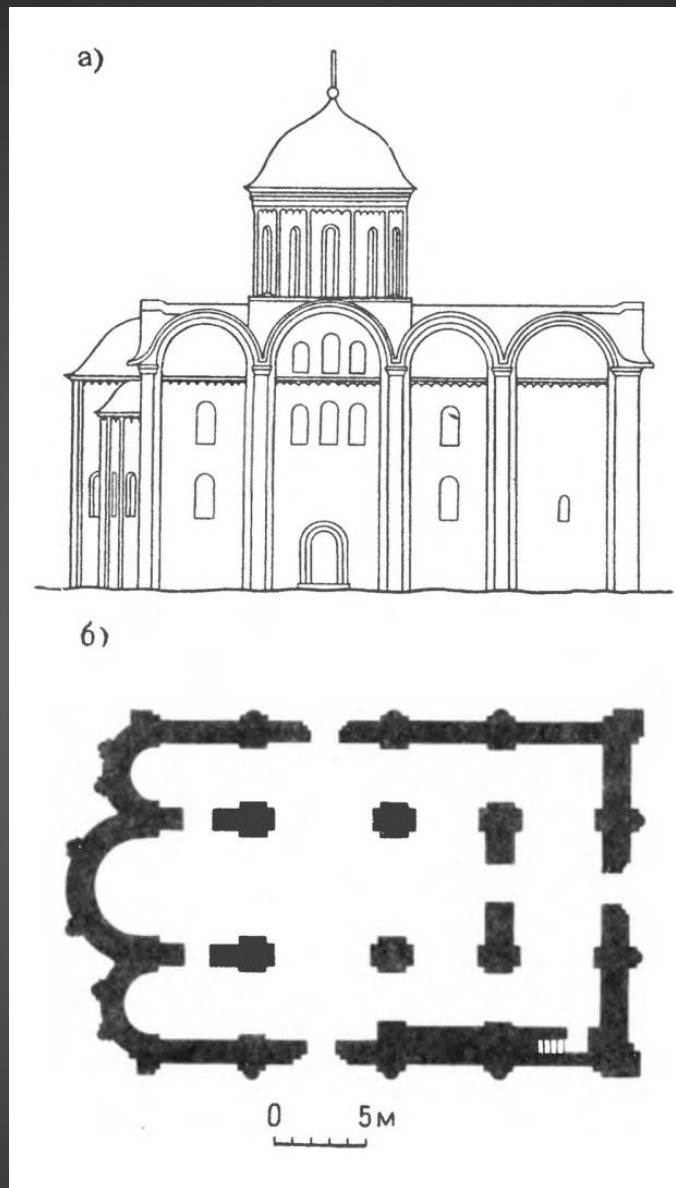
Успенский собор. Старая Рязань. Первая четверть XII в. Реконструкция и план.
