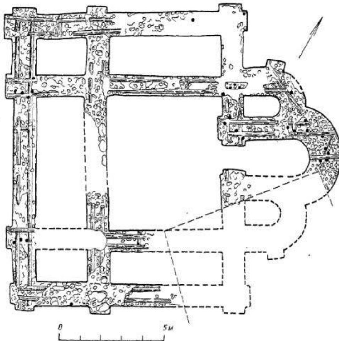
Церковь Андрея в Переяславле. План раскопанных фундаментов. По П.А.Раппопрту («Строительное производство Древней Руси X-XIII вв., 1993»).
