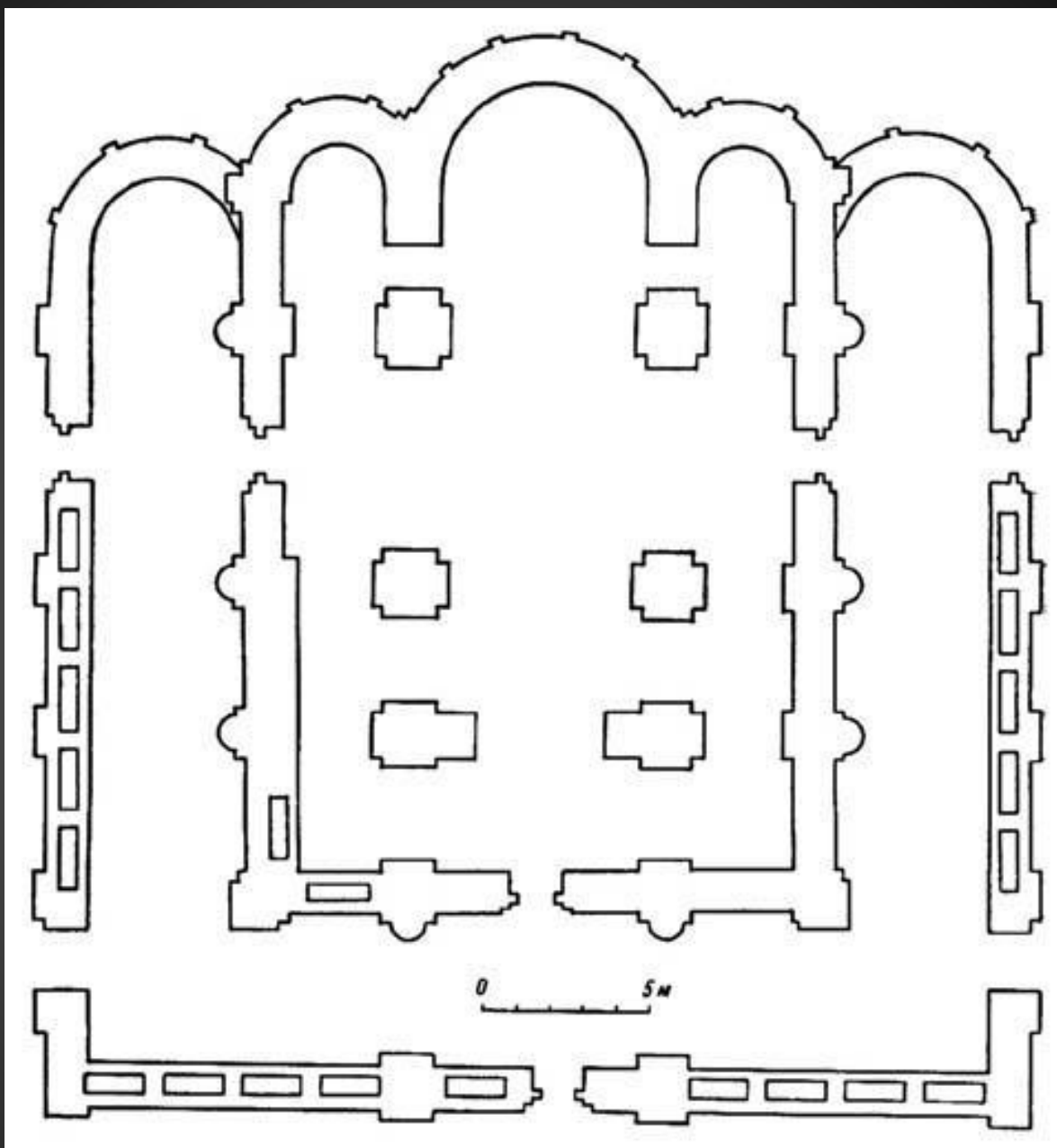
Собор Борисоглебского Смядынского монастыря. Смоленск. середина, XII в. План
