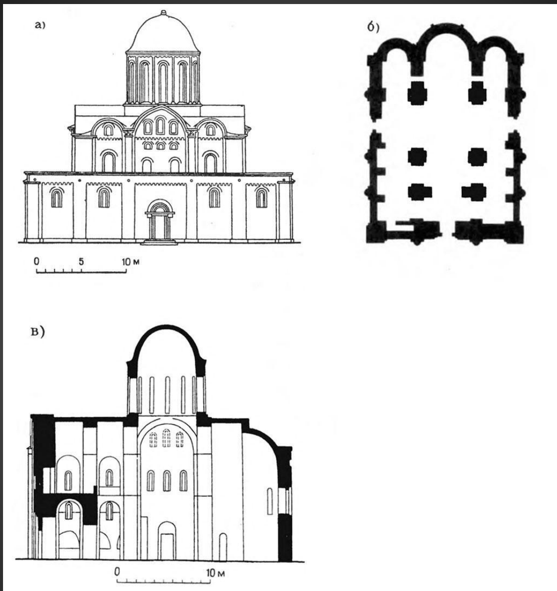
Борисоглебский собор. Чернигов. 20-е гг. XII в. План, разрез.
