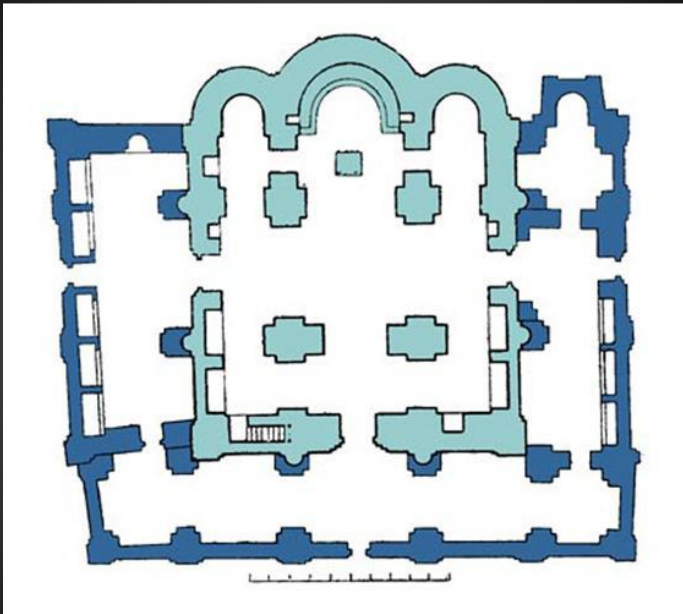
Церковь Петра и Павла. Смоленск. 1140—1150. План.
