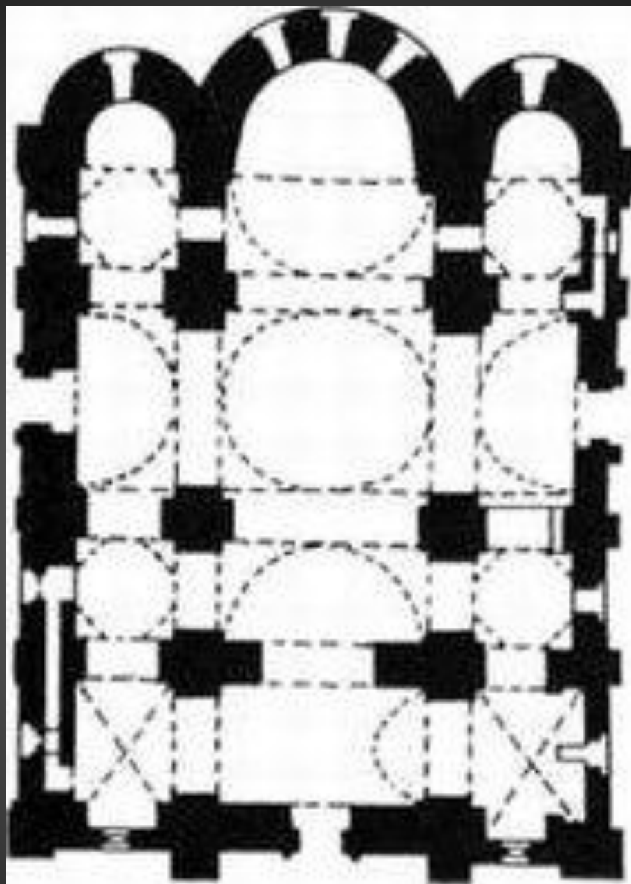
Кирилловская церковь. Киев. 40-е гг. XII в. План.
