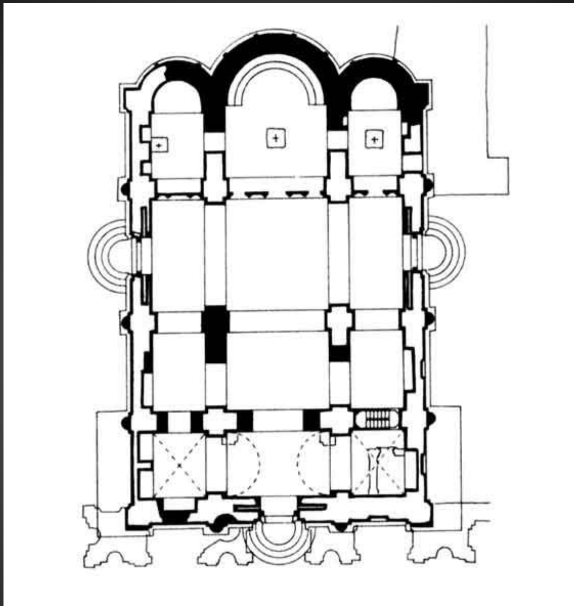
Успенский собор. Владимир-Волынский. 1160. План.
