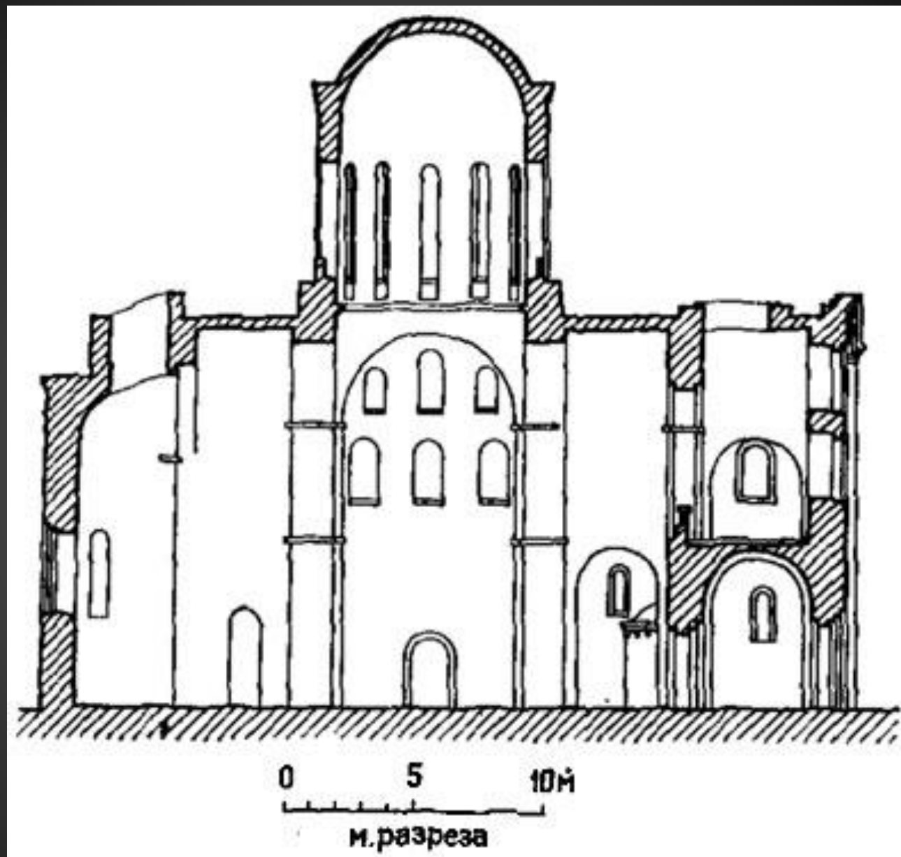
Успенский собор Елецкого монастыря. Чернигов. Разрез.
