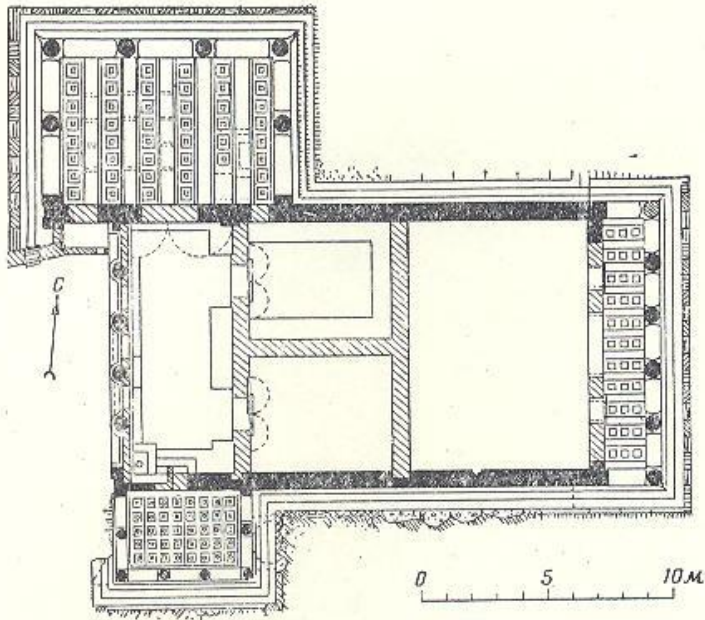
127. Эрехтейон в Афинском Акрополе, 421 — 407 гг. до н. э. План
