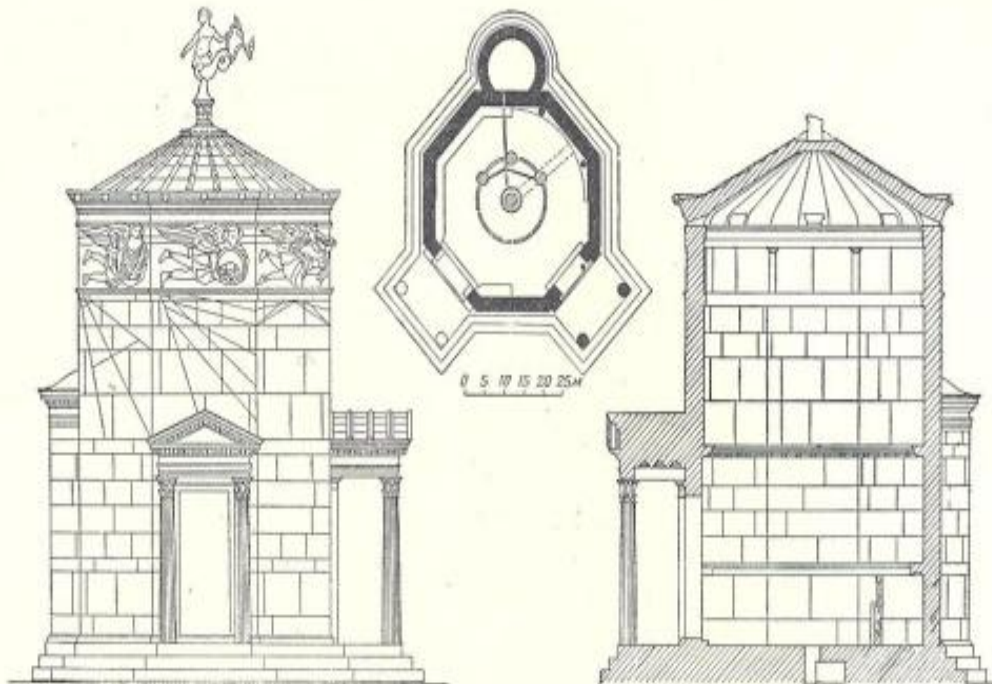
149. «Башня ветров» в Афинах, середина I в. до н. э. Фасад, план, разрез
