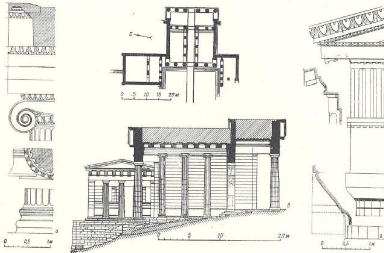
133. Пропилеи в Афинском Акрополе, 437 — 432 гг. до н. э. Арх. Миссикл. а—детали внутреннего дорического ордера; б — план; в — разрез (реконструкция); г — детали ордера восточного фасада
