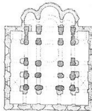
План
