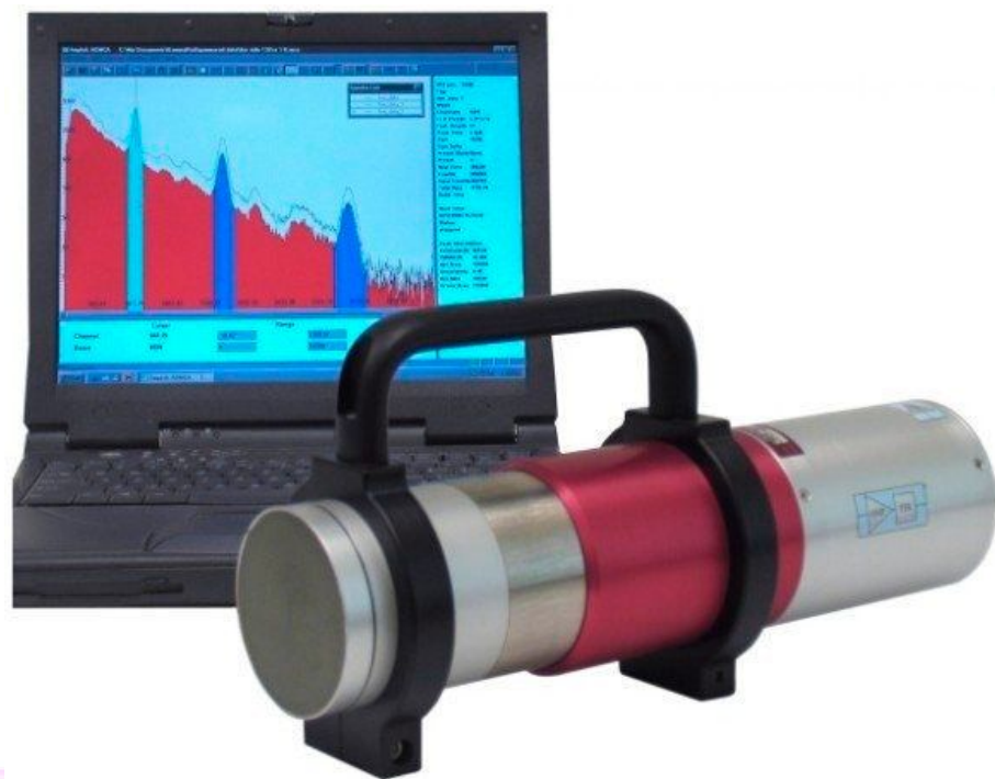
Гама-спектрометрія
