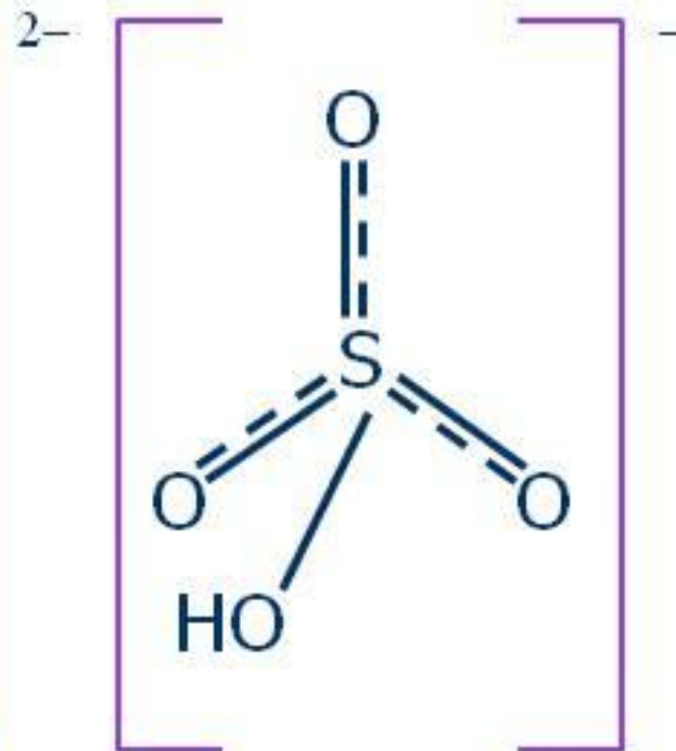
Гидросульфат-ион
