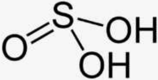
Сернистая кислота
