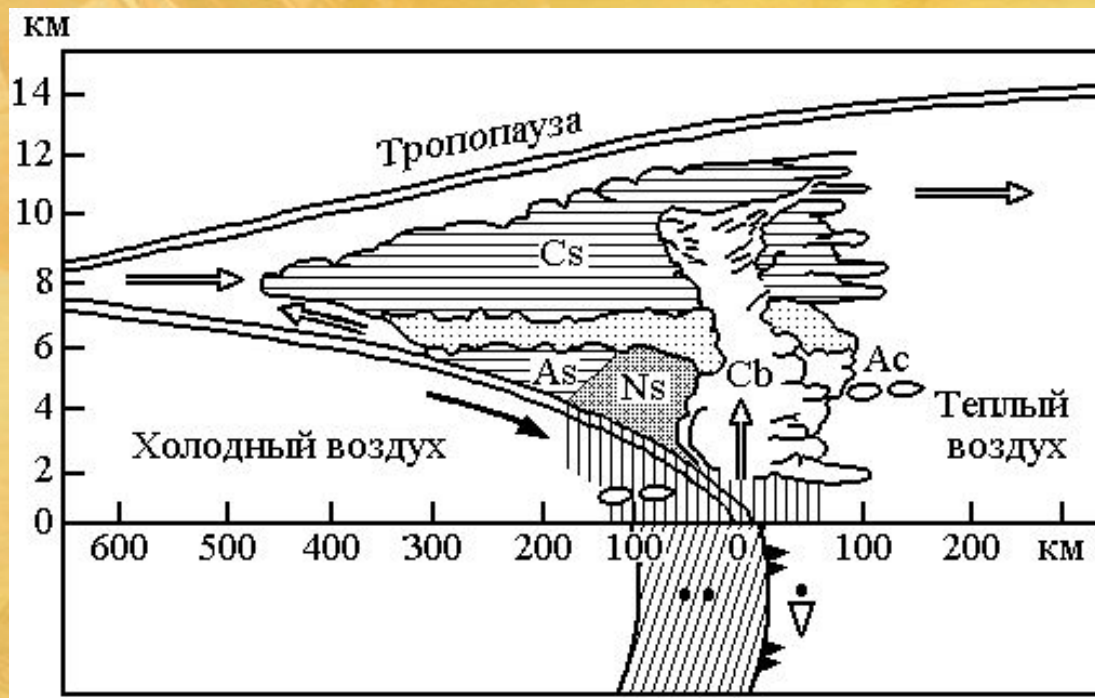
Холодный фронт в разрезе
