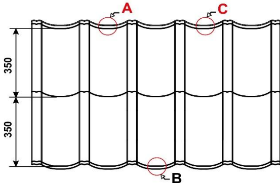
З'єднання листа
