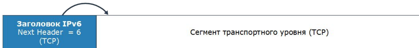
IPv6-пакет без расширенных заголовков
