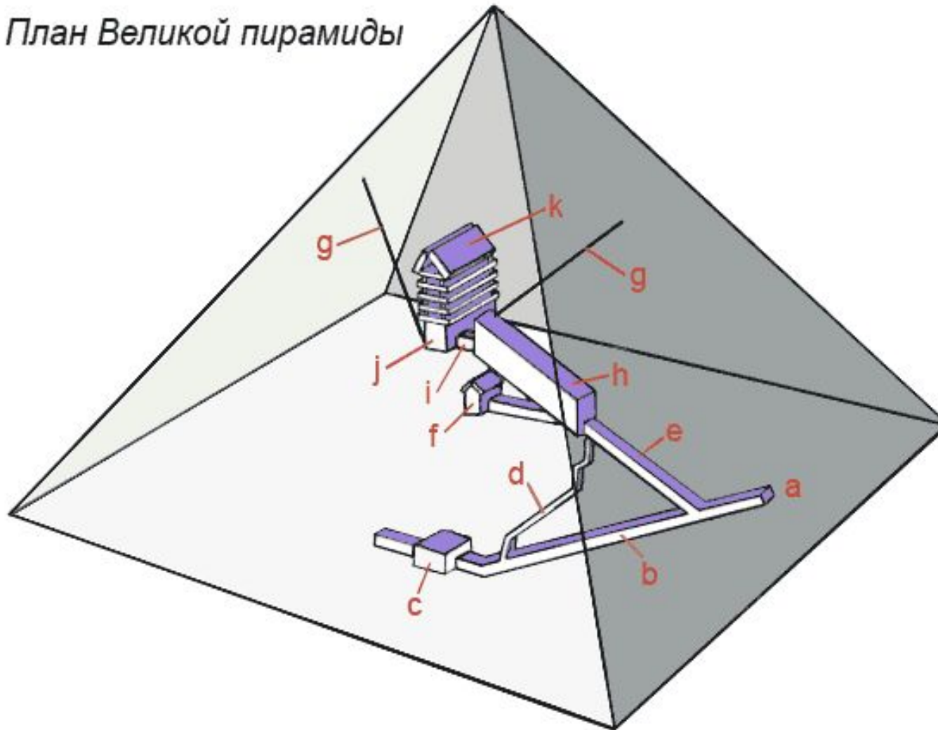
ВНУТРЕННЕЕ УСТРОЙСТВО ПИРАМИДЫ ХУФУ
