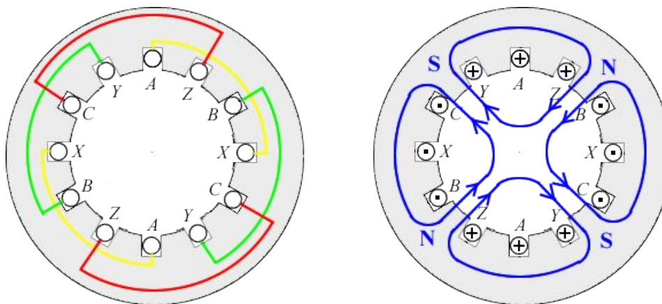
Четырехполюсная обмотка асинхронного двигателя ( p=2 )
