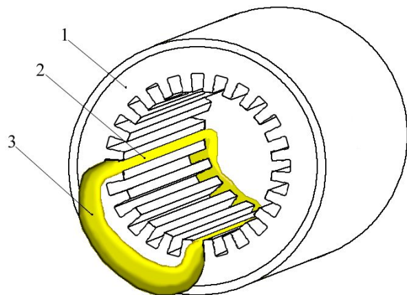
Катушка обмотки статора.
