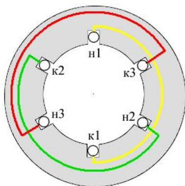
Расположение фаз трехфазной обмотки статора в пазах
