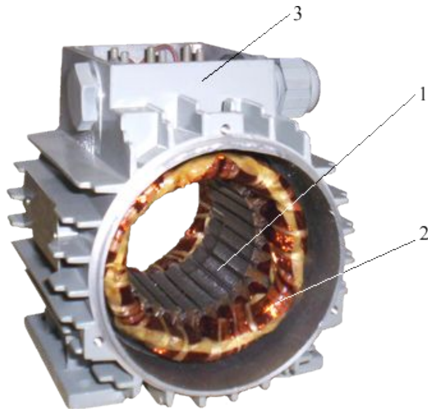
Статор асинхронного двигателя АОЛ-012/4.
