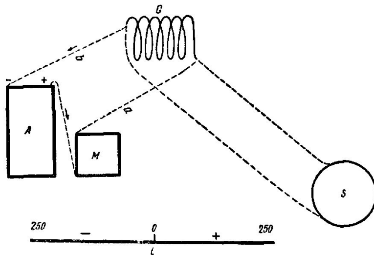
G — гальванометр, A — аккумулятор, S — шунт, M — реостат, S — шкала.
