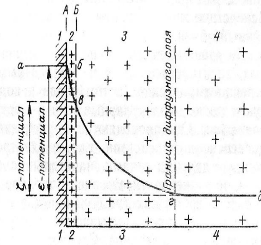
Рис. IV-21. Схема двойного электрического слоя.
