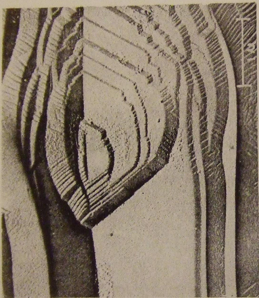
Struktura krystalu bariem titanátu v elektrovém mikroskopu
