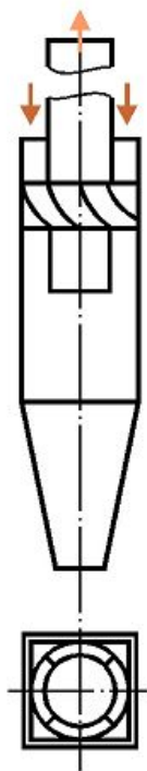
С восьмилопастными лопатками безударного входа (тип БЦ)
