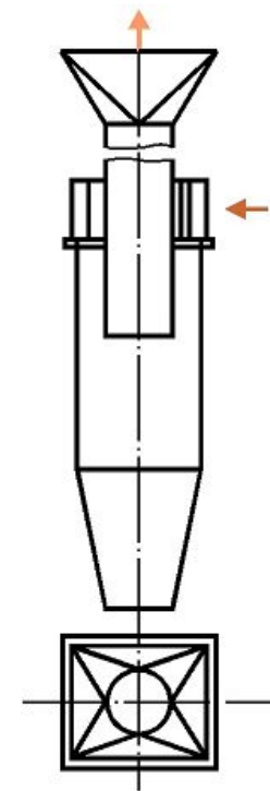
С тангенциальным четырехзаходным завихрителем (тип БЦ-512)
