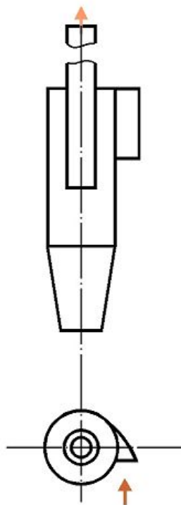
С полуэллиптическим входом (тип БЦУ)
