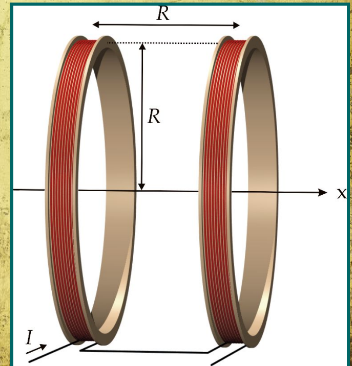
пара катушек Гельмгольца
