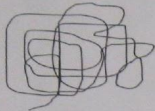
ГЕНОМНАЯ ДНК
