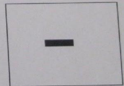
АВТОРАДИОГРАФИЯ
