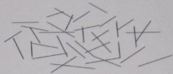
10^6 ФРАГМЕНТЫ ДНК
