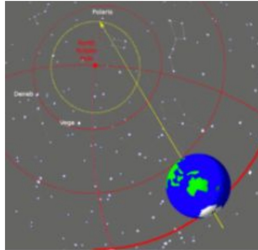
Прецессия земной оси вокруг Северного полюса эклиптики
