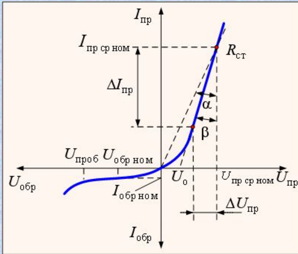
Вольт-амперная характеристика выпрямительного диода
