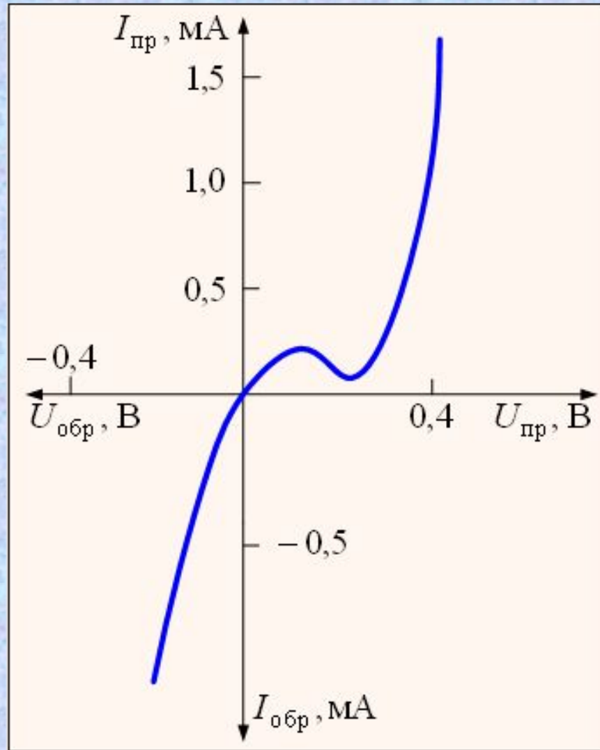
Вольт-амперная характеристика обращенного диода
