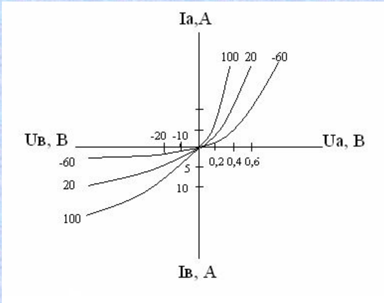
Вольт-амперная характеристика диода Шоттки
