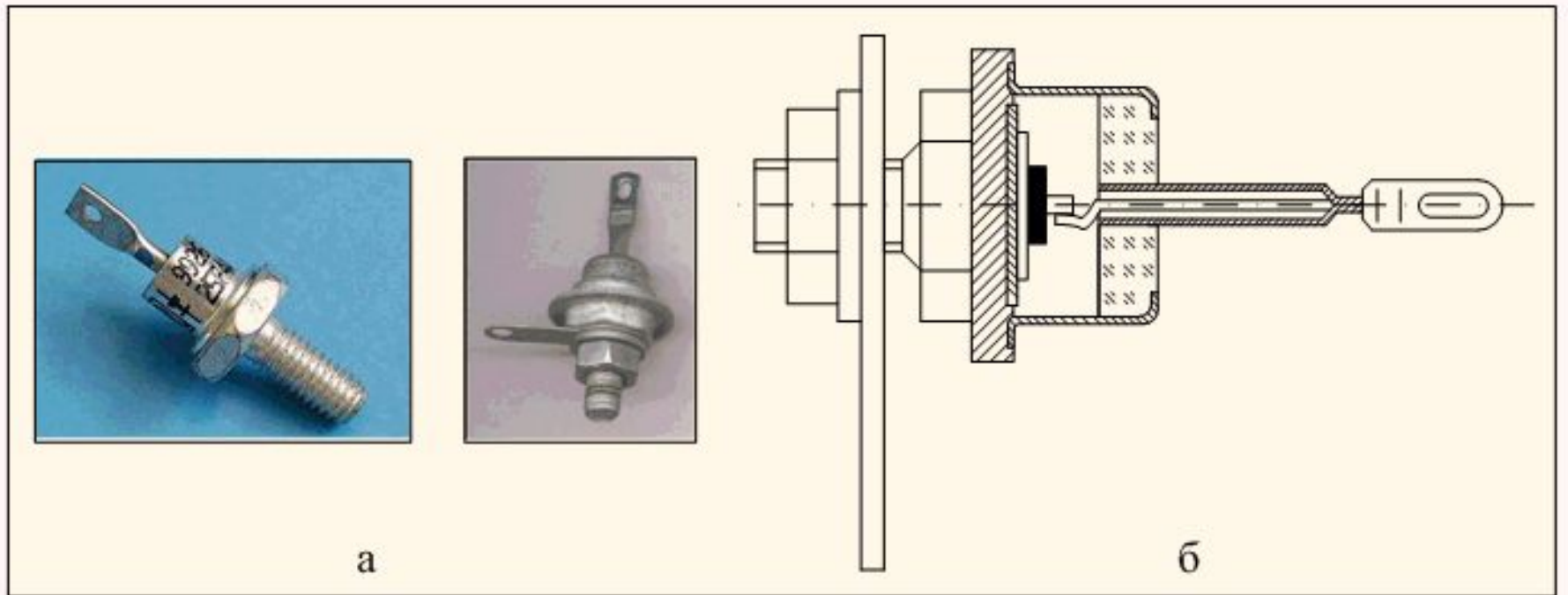
Вид (а) и конструкция (б) мощного кремниевого выпрямительного диода
