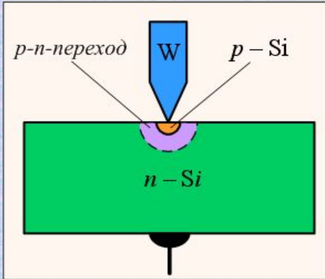
Структура точечного диода
