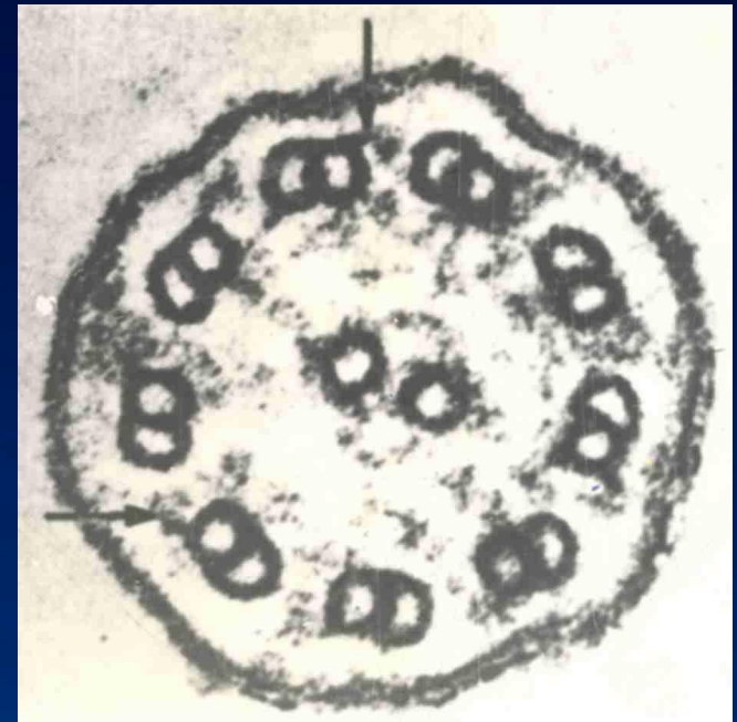
Поперечный срез реснички
