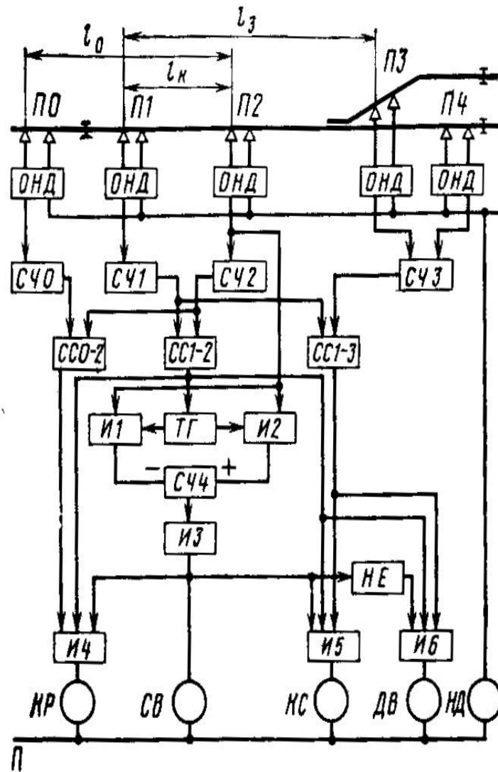
Рис. 10.16. Структурная схема комплексного контроля головной стрелки УКГЗ
