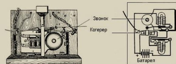
Внешний вид и схема радиоприемника А.С. Попова
