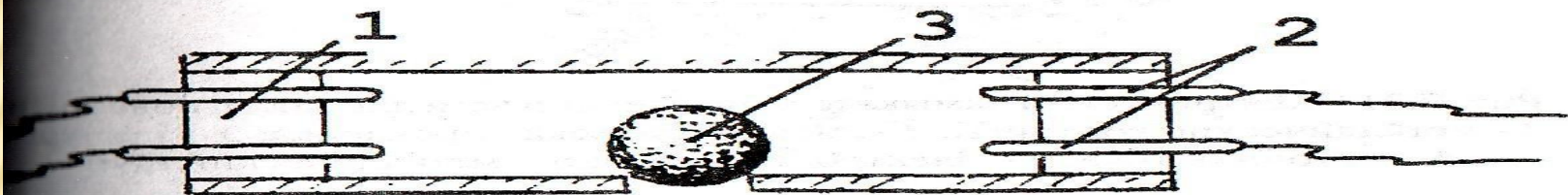
Рис. 7.29 Электрический замыкатель гравитационной конструкции. 1 – диэлектрический корпус; 2 – металлические контакты; 3 – металлический шарик.
