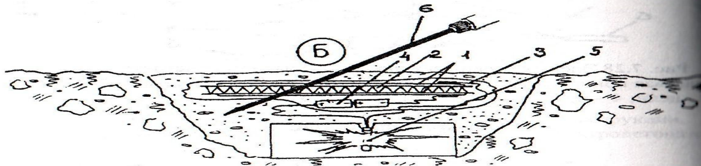
Рис. 7.31 Электрический замыкатель по степени замедления мгновенный. 1 – металлические контакты; 2 – диэлектрическая прокладка; 3 – провод; 4 – источник тока; 5 – электродетонатор; 6 – металлический шуп.
