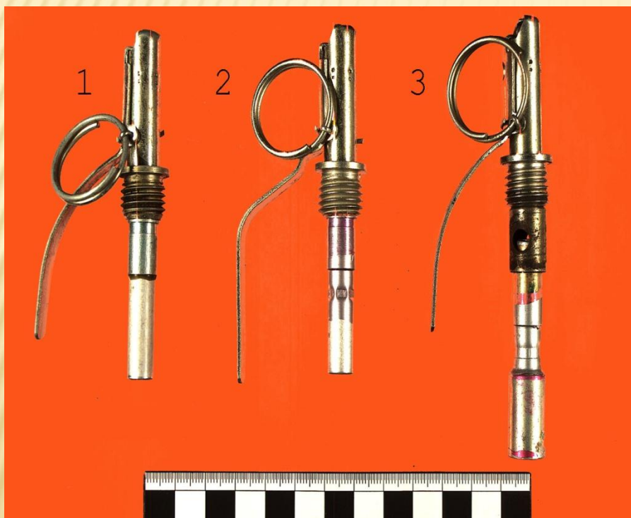
Взрыватель УЗРГМ-2
