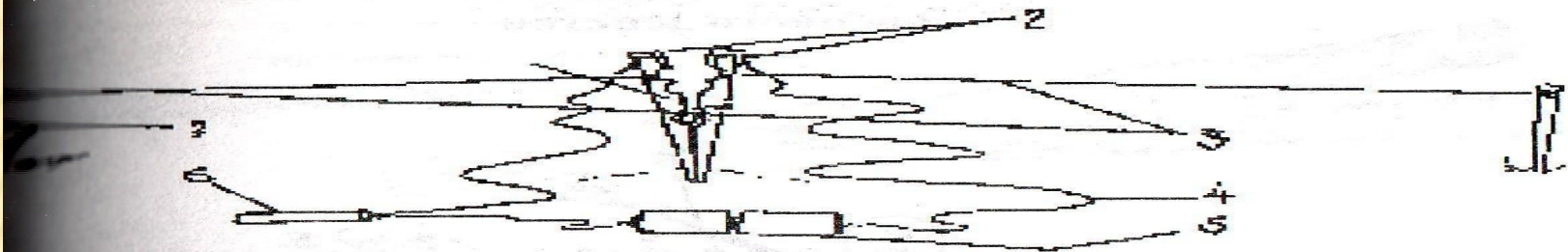
Рис. 7.28 Электрический замыкатель обрывной конструкции. 1 – бьющая прищепка; 2 – металлические контакты; 3 – обрывной датчик цели; 4 – провода; 5 – источник тока; 6 – электродетонатор.
