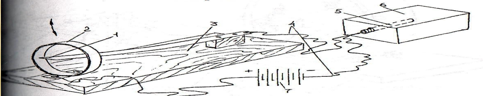
Рис. 7.30 Электрический замыкатель вибрационной конструкции. 1, 2 – металлические контакты; 3 – основание; 4 – провода; 5 – электродетонатор; 6 – заряд ВВ; 7 – источник тока.
