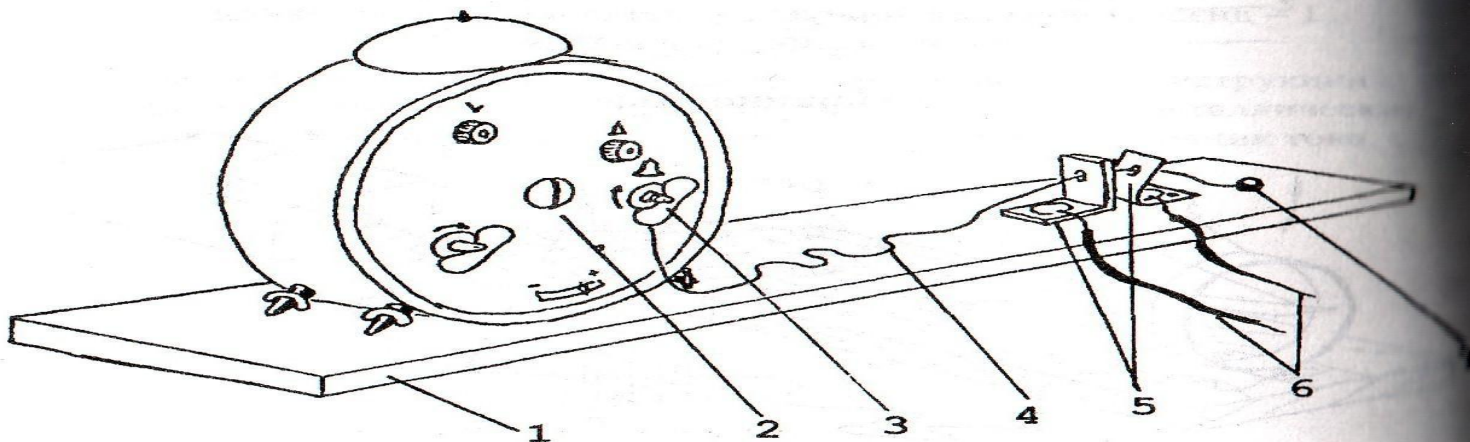
Рис. 7.32 Электрический замыкатель замедленного действия часовой. 1 – основание; 2 – будильник; 3 – привод заводного механизма; 4 – нить; 5 – металлические контакты; 6 – провода; 7 – груз.
