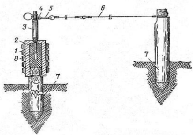
Противопехотная мина ПОМЗ-2М: 1 — корпус; 2 — заряд ВВ — 75-г. тротиловая пашка; 3 — взрыватель МУВ-2; 4 — Р-образная боевая чека; 5 — карабин с отрезком проволоки; 6 — проволоочная растяжка; 7 — колышки; 8 — завал МД-6М
