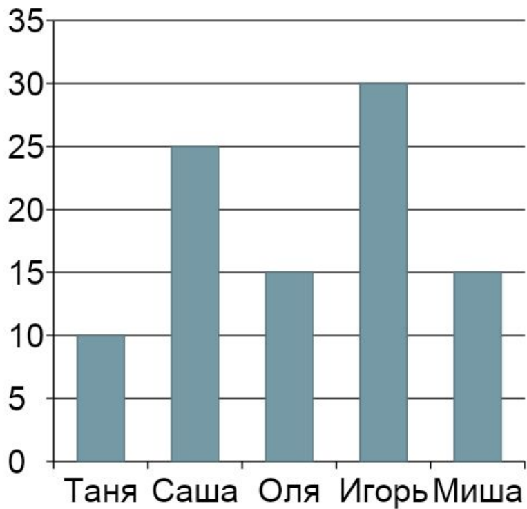
Столбчатая диаграмма
