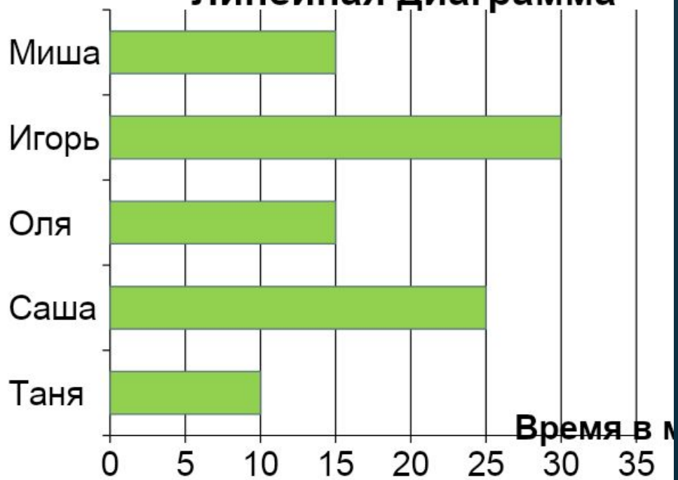
Линейная диаграмма
