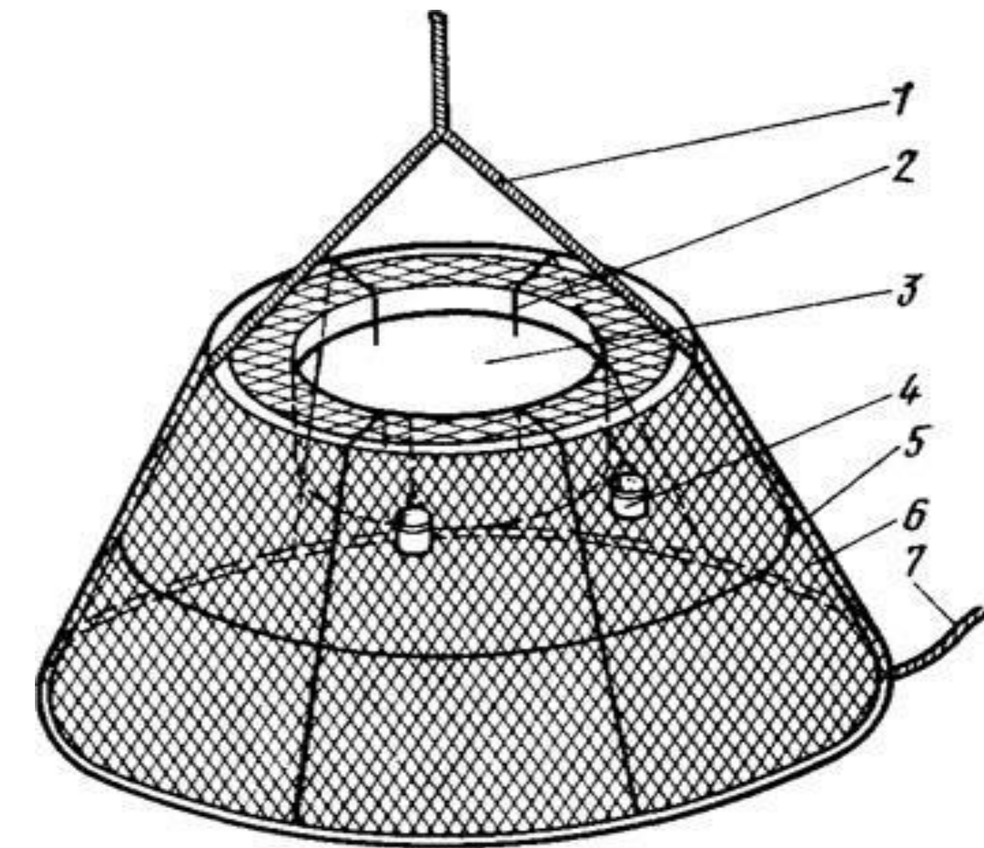
Рис. 8. Строение крабовой ловушки
