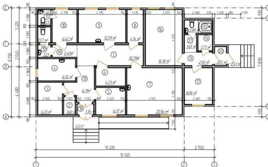
План этажа
