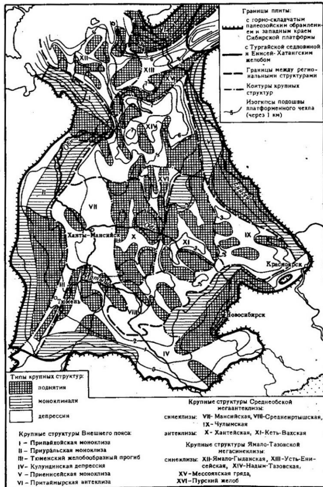
Рис. 3. Тектоническая схема Западной Сибири (по И. И. Нестерову)
