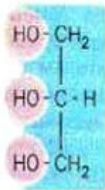
глицерин
