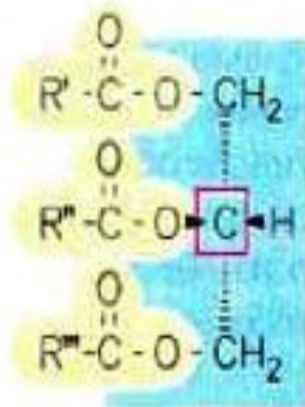
триацилглицерин (жир)
