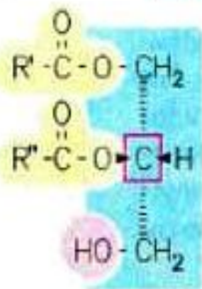
диацилглицерин
