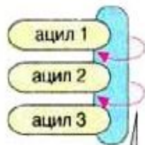
триацилглицерин (жир)
