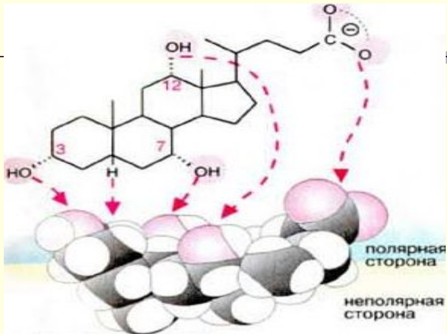
Холевая кислота
