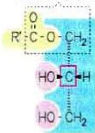
моноацилглицерин
