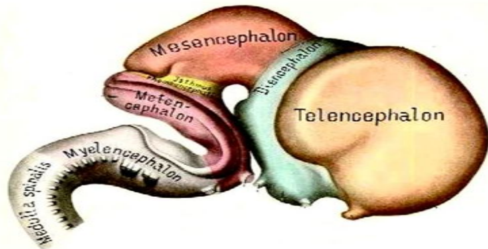
пятипузырная стадия
