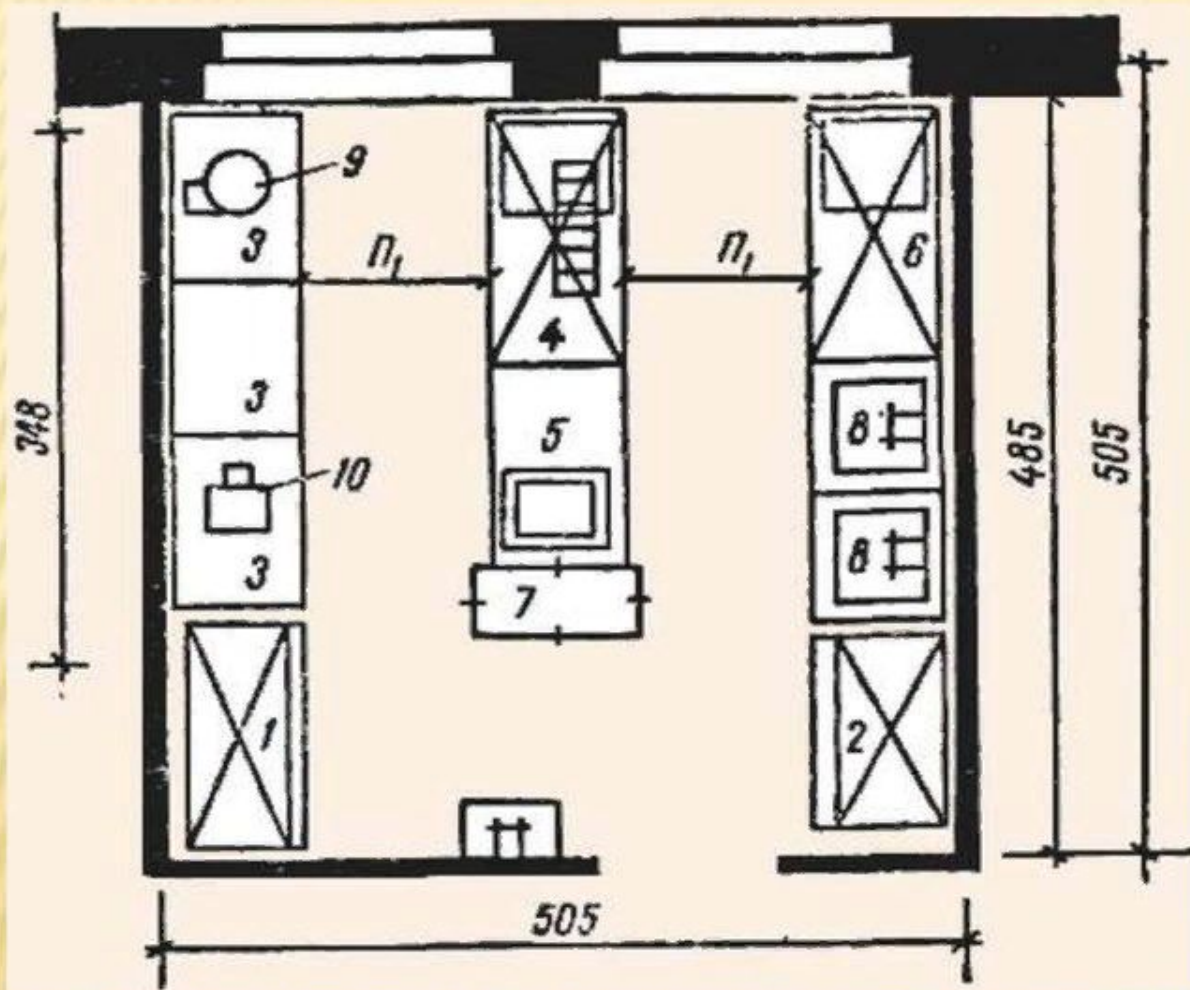
План холодного цеха общедоступной столовой
