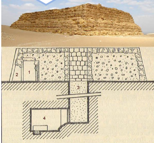
1 - МОЛЕЛЬНЯ; 2 - СЕРДАБ; 3 - ШАХТА; 4 - КАМЕРА С САРКОФАГОМ.
