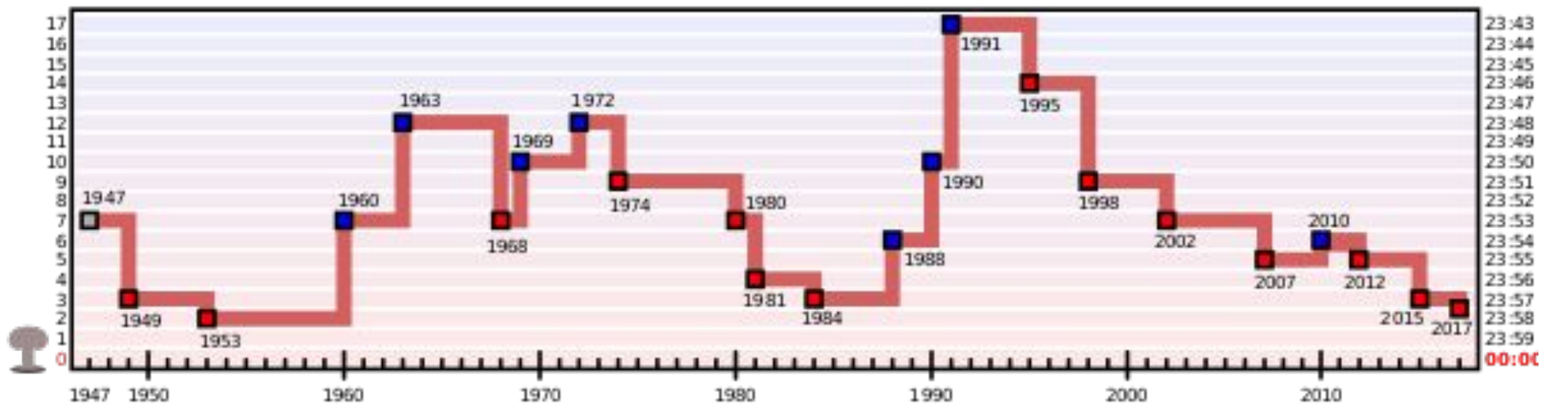
Часы судного дня: число минут до полуночи, 1947-2017
