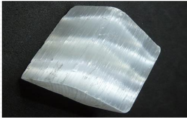
Селенит
