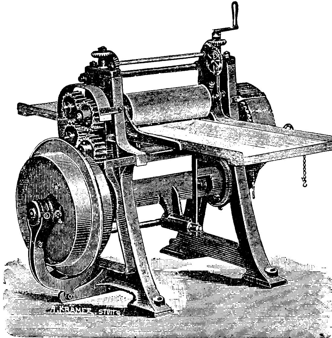
Фиг. 3. Вальцы со столикомъ для прокатки листовъ.
