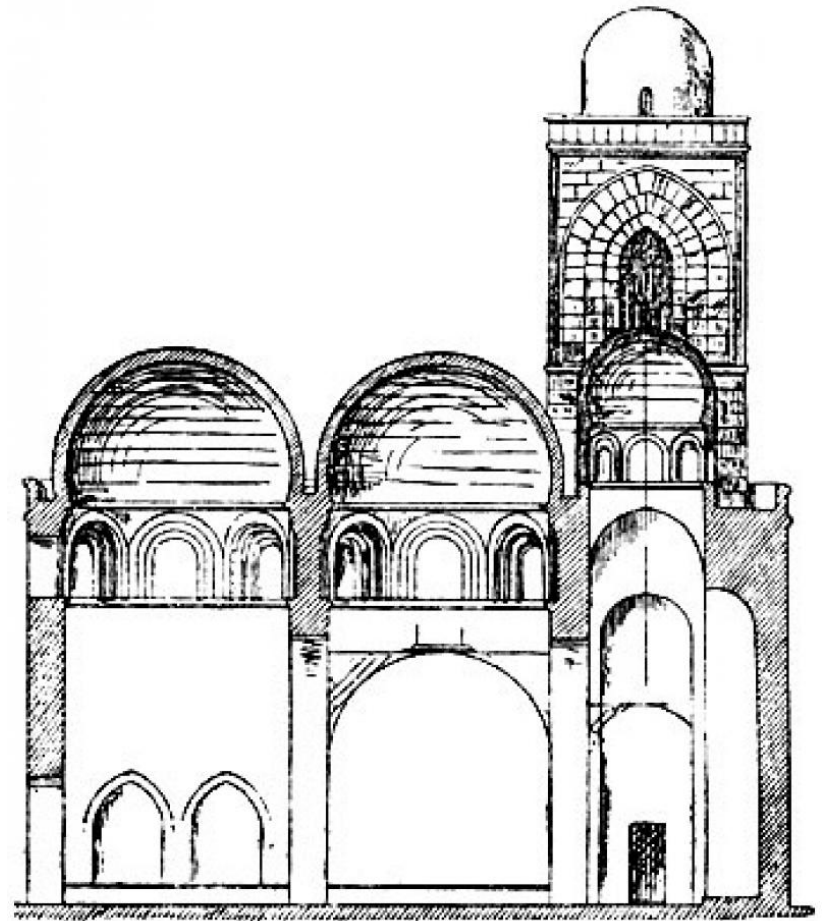
Церковь Сан Джованни дельи Эремити в Палермо. Продольный разрез.
