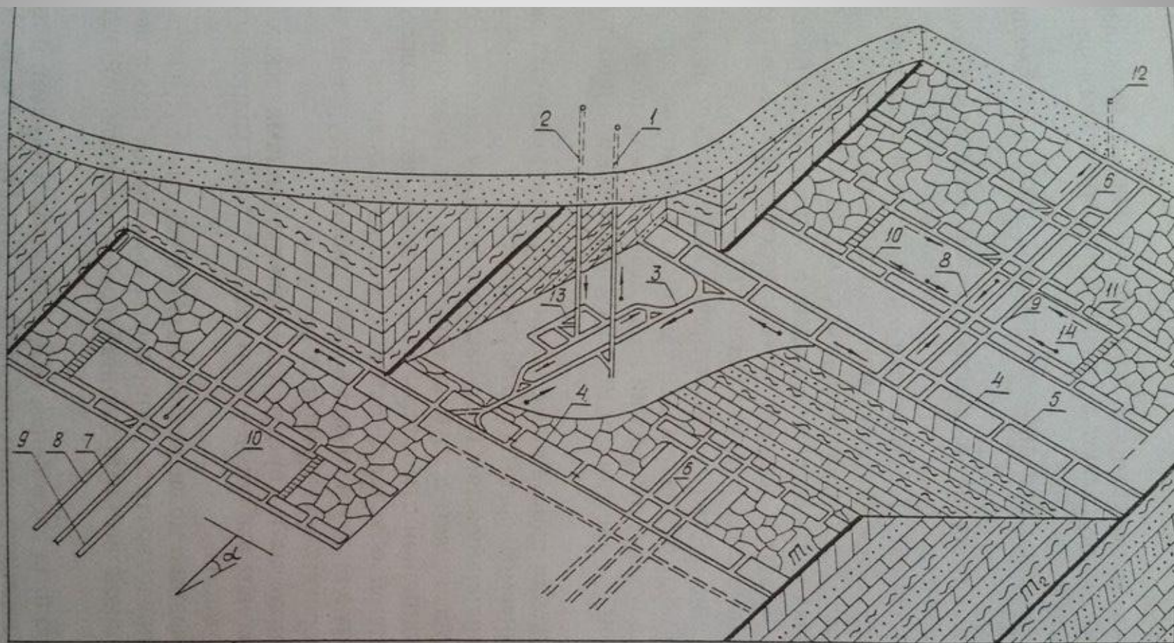
Рис. 1.1. Схема угольной шахты:
