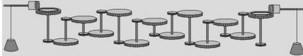
Эскиз счетной машины Леонардо да Винчи
