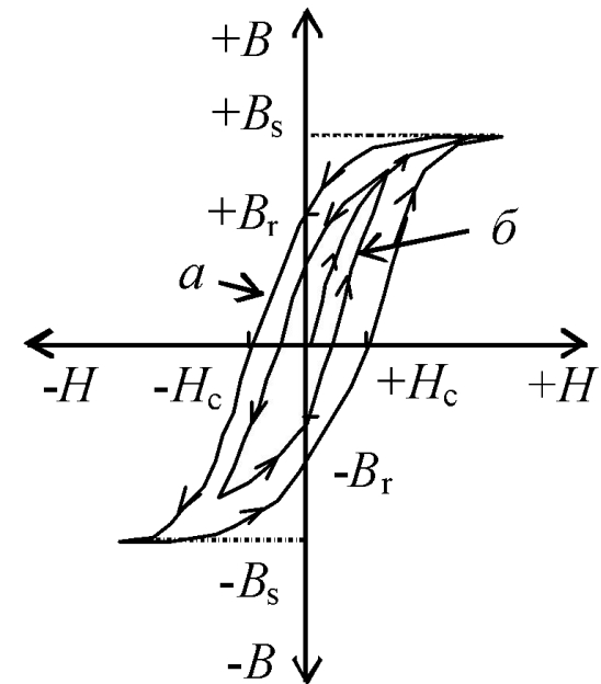
Рис. 3.13. Предельная - a и частная - б кривые намагничивания при циклическом перемагничивании
