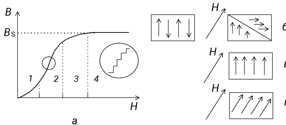
Рис. 3.12. Основная (начальная) кривая намагничивания ферромагнетика a ; условные изображения структуры доменов на различных участках кривой намагничивания: б - необратимое смещение доменных границ на участке 2; в - процесс вращения на участке 3; г - ориентация магнитных моментов вдоль поля на участке 4
