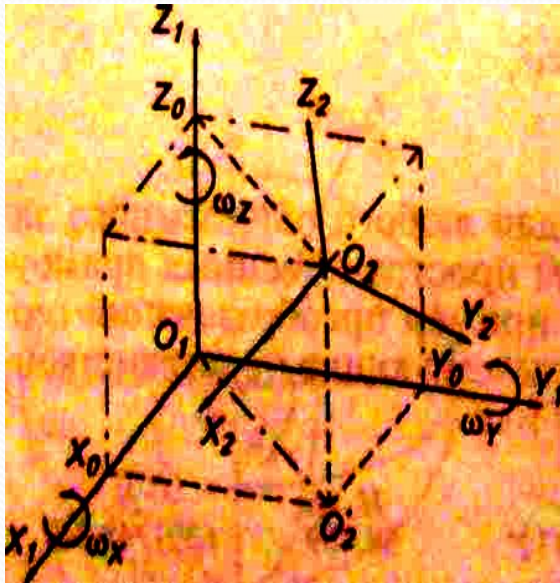
Рис. 1.4. Параметры связи двух пространственных систем прямоугольных координат
